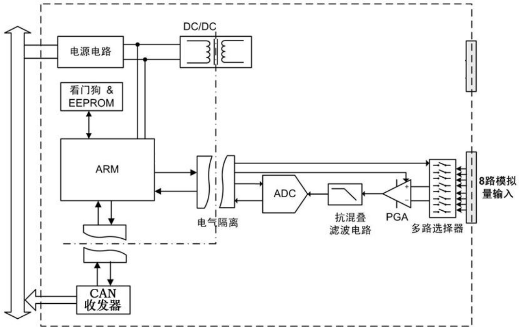
图 1.2 C-4008 原理框图
